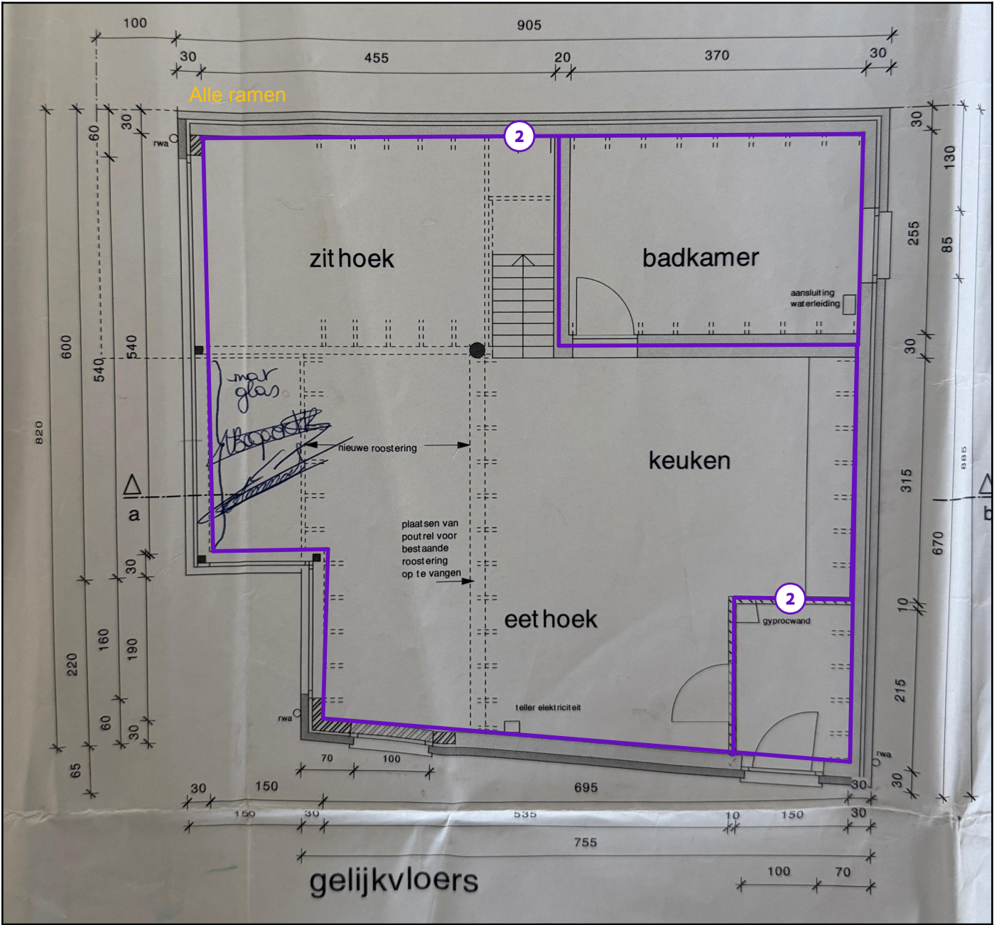
Legende van plan 1.1: Gelijkvloers muren
