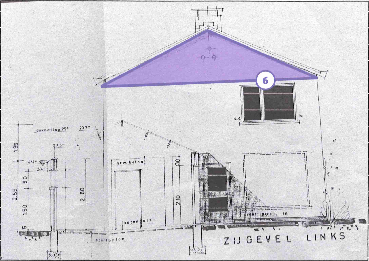
Legende van plan 1.3: Zijgevel links
