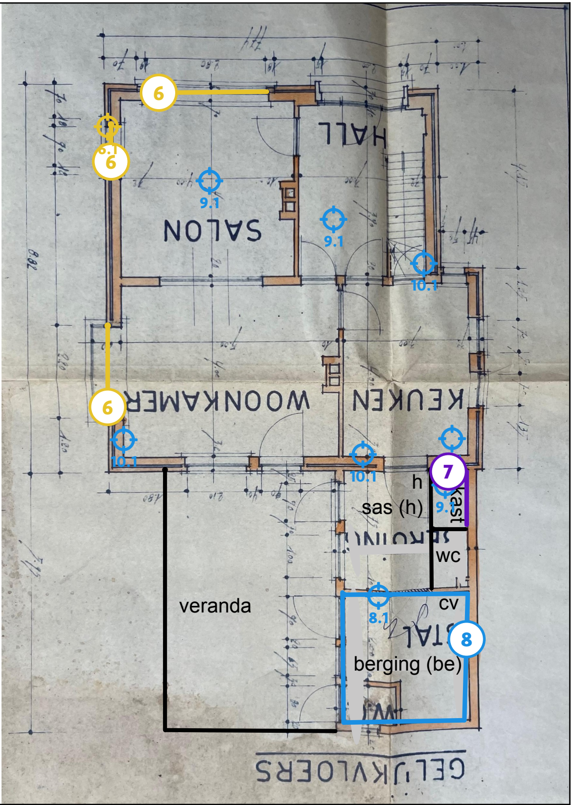
Legende van plan 1.3: Gelijkvloers woning
