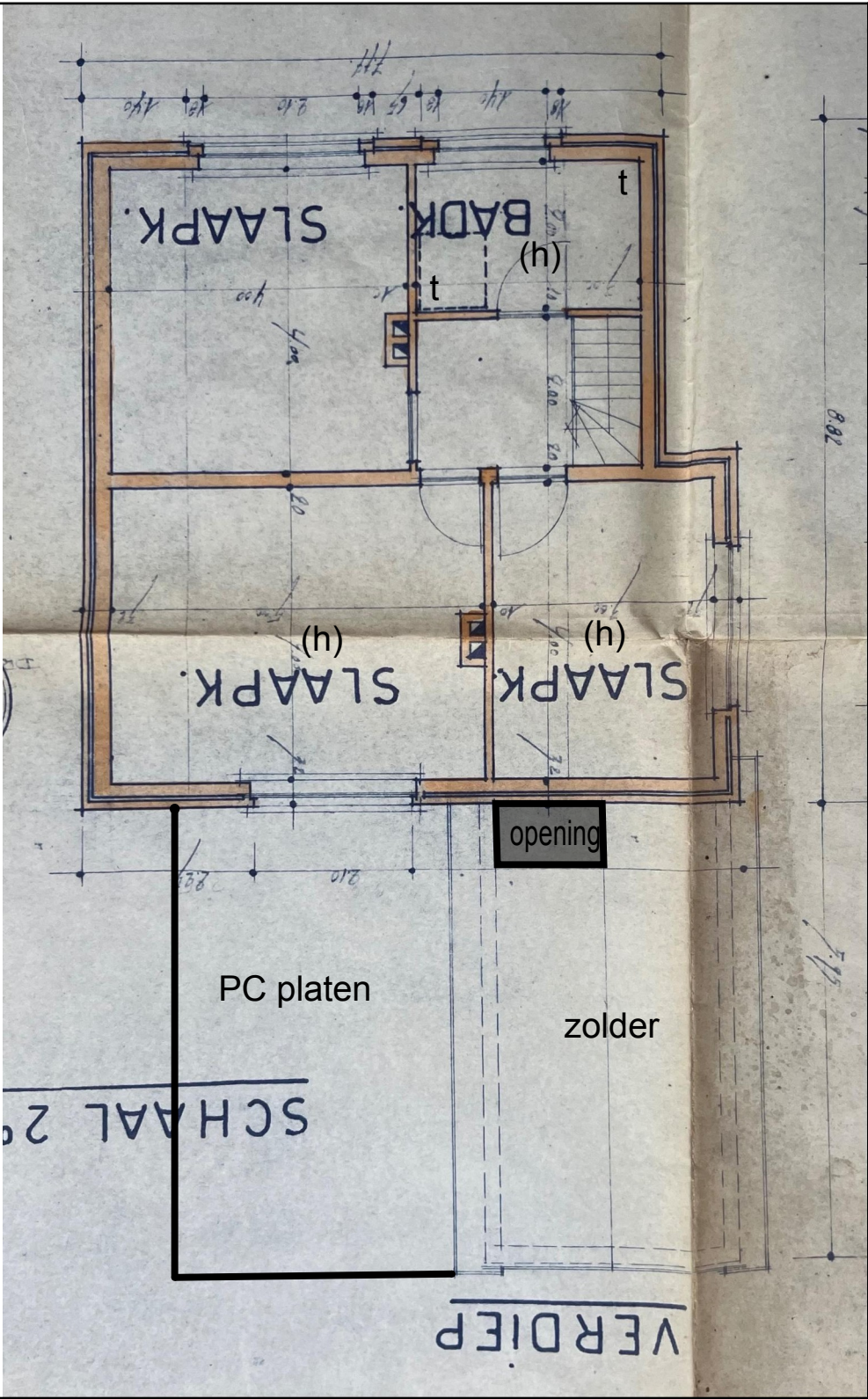
Legende van plan 1.5: 1ste verdieping woning
