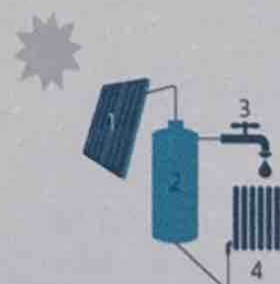
1. Zonnecollector | 2. Opslagvat zonneboiler | 3. Sanitair warm water | 4. Afgifte-element voor ruimteverwarming (optioneel)
