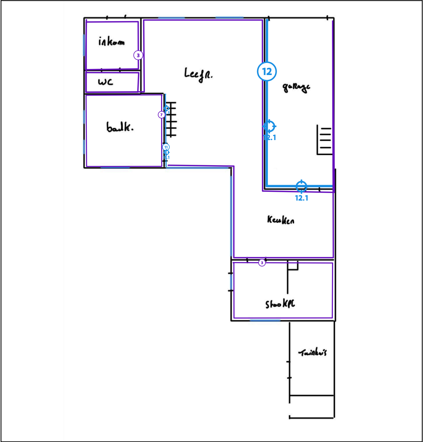
Legende van plan 1.2: Gelijkvloers wanden
