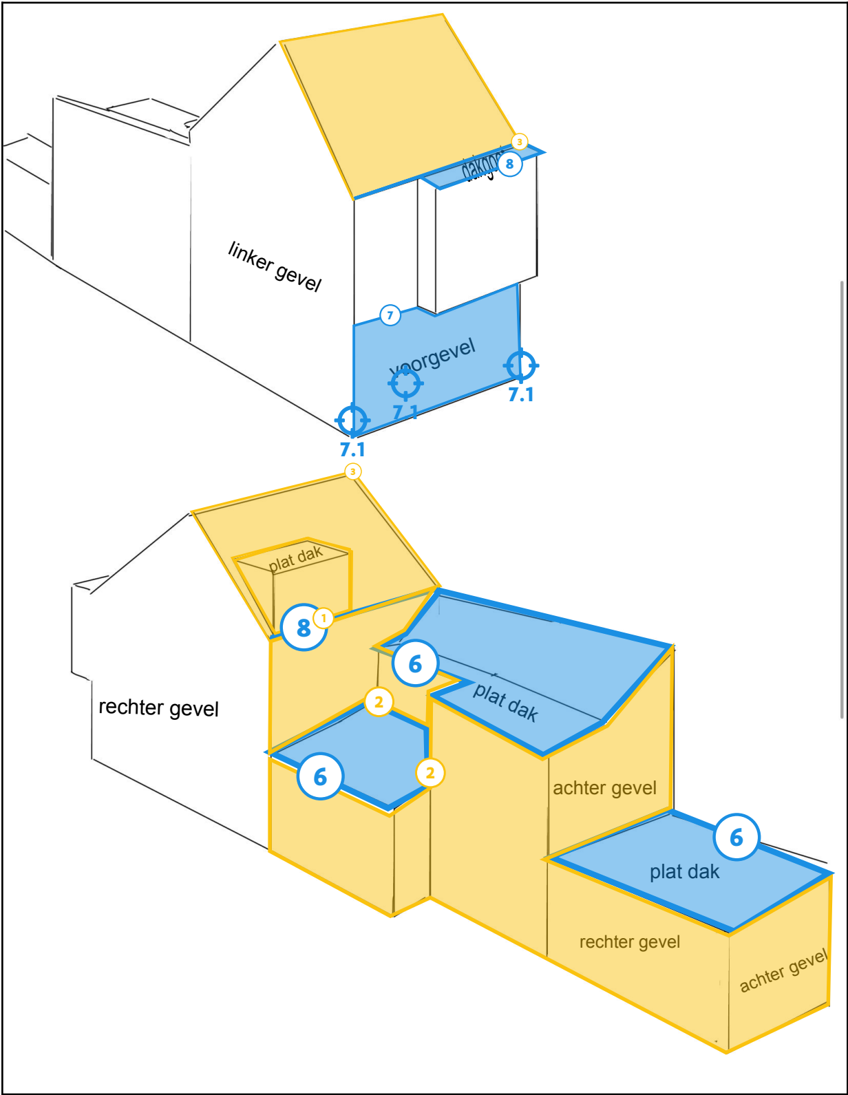
Legende van plan 1.1: Zij aanzichten
