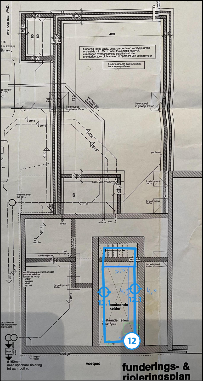
Legende van plan 1.15: Kelder
