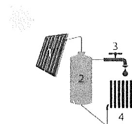
1 Zonnecollector | 2 Zonneboiler | 3 Opslagvat voor warm water | 4 Radiator voor verwarming
